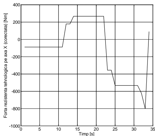
Fig. 5.16. Forța rezistentă tehnologică pe axa X, corectată
