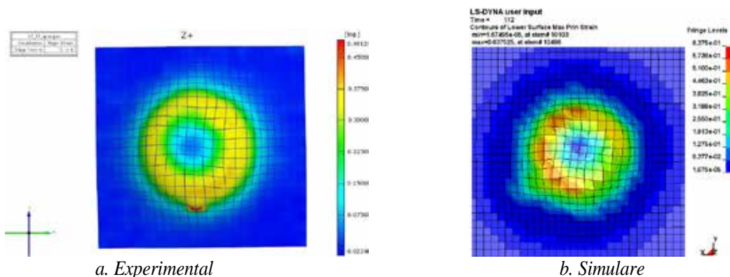
Fig. 4.66. Deformațiile principale maxime pentru piesele de tip trunchi de con 2507_TC_10_55_SAC_240
