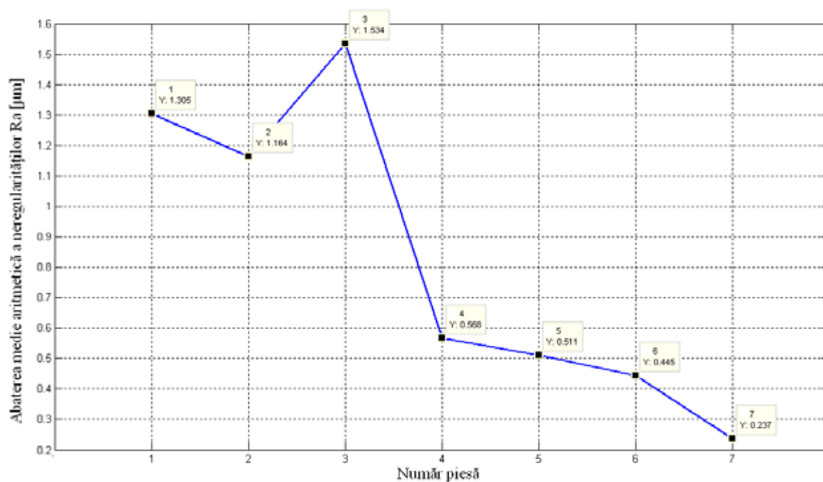
Fig. 4.88. Abaterea medie aritmetică a neregularităților R_a [ \mu\text{m} ]
