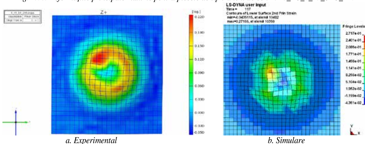
Fig. 4.69. Deformațiile secundare maxime pentru piesele de tip trunchi de con 2518_TC_6_45_SAC_240
