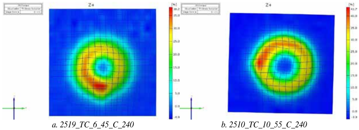
Fig. 4.47. Distribuțiile subțierii relative pe piesele trunchi de con, traiectorie circulară
