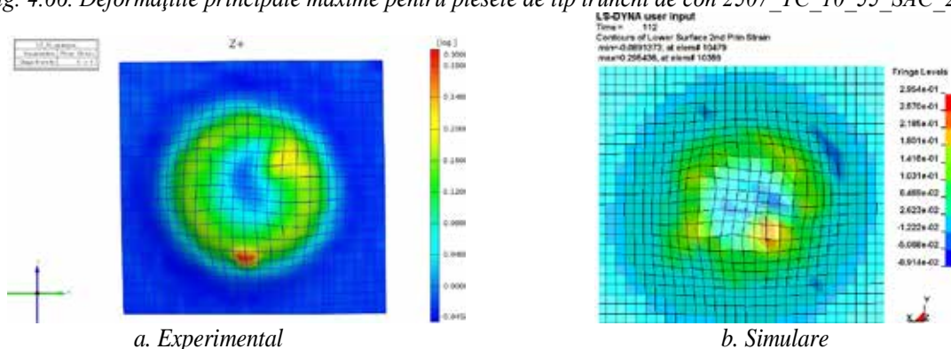
Fig. 4.67. Deformațiile secundare maxime pentru piesele de tip trunchi de con 2507_TC_10_55_SAC_240
